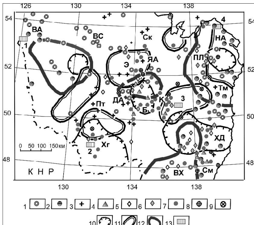
Рис. 8. Прогнозирование рудоперспективных площадей в Среднем Приамурье по аномалиям m_z -параметра: 1–9 – месторождения и крупные рудопрооявления [12]: золота (1), золото-серебряные (2), молибдена (3), меди (4), вольфрама (5), олова с вольфрамом (6), 7 – олова, 8 – полиметаллов, 9 – сурьмы; 10–12 – районы, перспективные для поисков: олова (10), вольфрама и полиметаллов (11), золота (12); 13 – горно-добывающие предприятия. Обозначения рудных районов: ВА – Верхне-Амурский, ВС – Верхне-Селемджинский, Ск – Селигканский, НА – Нижне-Амурский, ПЛ – Пильда-Лимурийский, ЯА – Ям-Алинский, Э – Эзопский, ДА – Дусе-Алинский, Б – Баджалский, Пт – Притуранский, К – Комсомольский, Тм – Тумнинский, ХД – Хуту-Джаурский, ВХ – Верхне-Хорский, См – Самаргинский. Обозначения добывающих предприятий: 1 – Покровское, 2 – Хинганское, 3 – Комсомольское, 4 – Многовершинное
