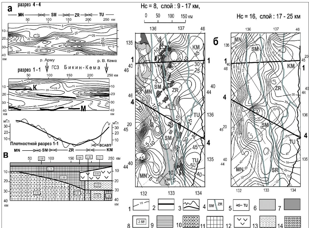
Рис. 5. Формализованный «реологический» (а) и плотностной (б) разрезы земной коры Сихотэ-Алиния; карты-срезы 3D-модели m_z -параметра (б):
