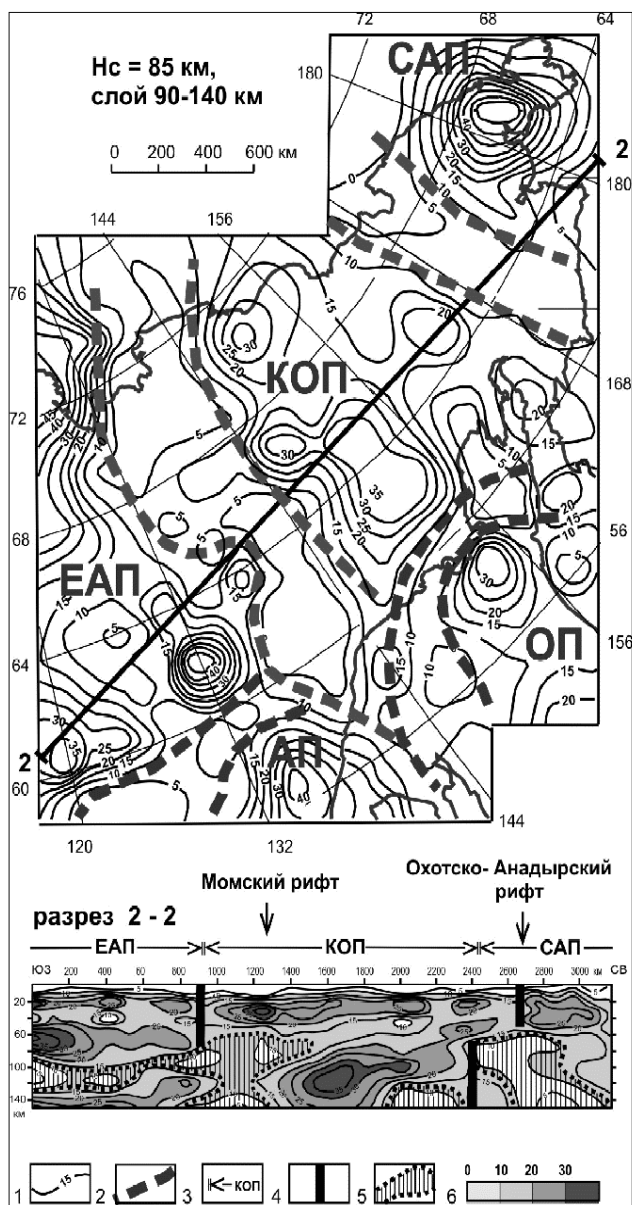
Рис. 1. Астеносфера и плиты Северо-Восточной Азии:
