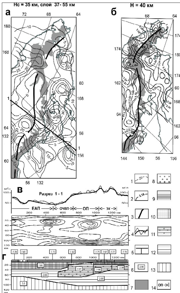
Рис. 3. Аномалии нормированной сферической плотности (а) и плотности (б) в основании Охотско-Чукотского вулканического пояса; формализованный по \mu_z -параметру (в) и плотностей (г) разрезы:
