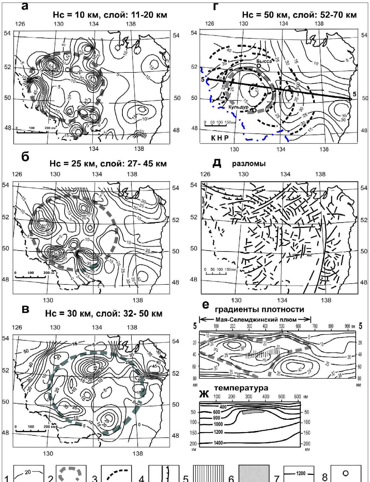
Рис. 7. Глубинная структура Мая-Селемджинского плюма: карты-срезы объемной модели \mu_z -параметра (а-г), разломы (д), градиентный (е) и температурный (ж) разрезы
