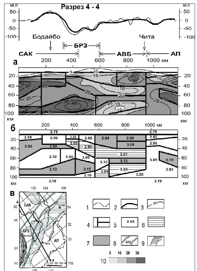
Рис. 4. Глубинное строение Байкальской рифтовой зоны в разрезе 4-4; распределение \mu_z -параметра (а), плотностной разрез (б) и структурная схема (в):
