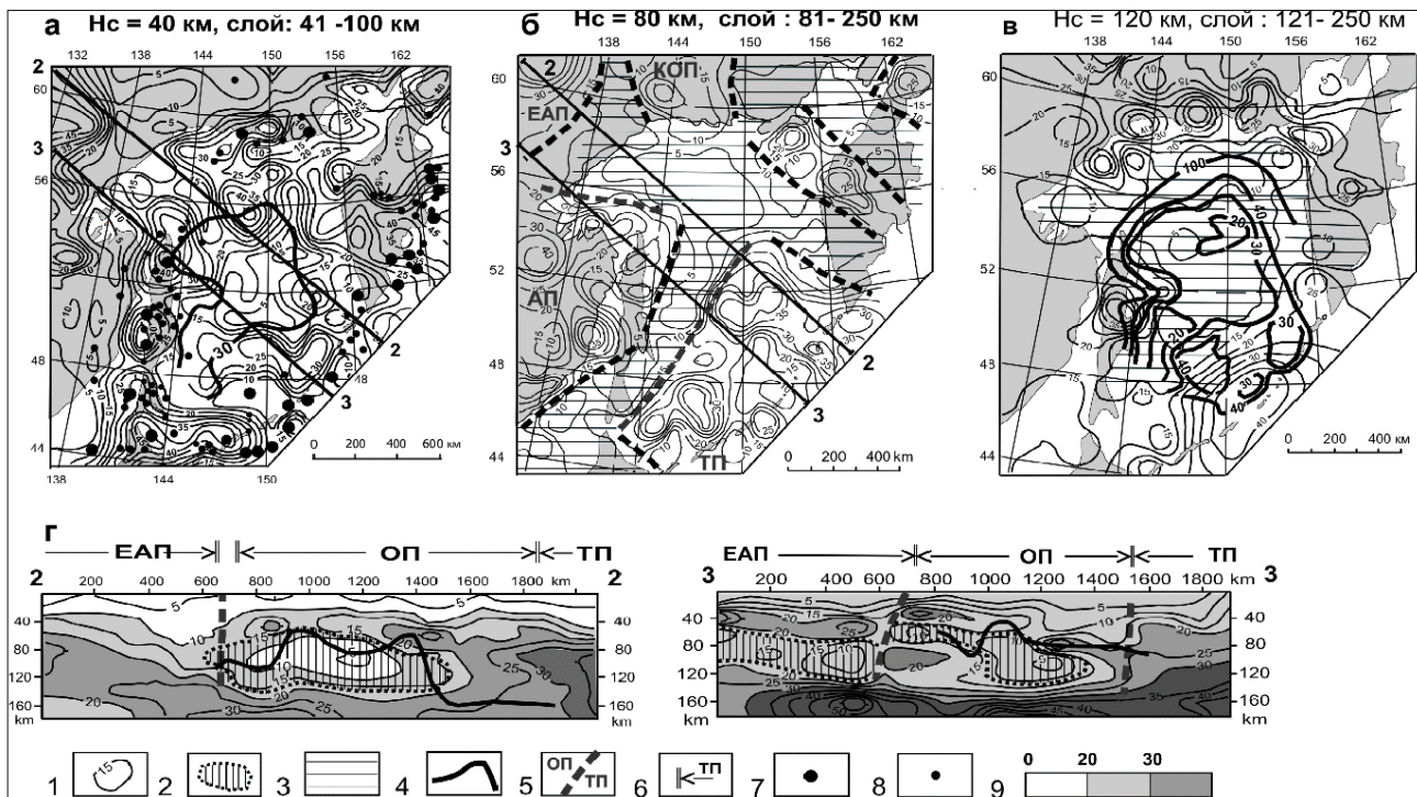
Рис. 2. Астеносфера и плиты Охотоморского региона:
